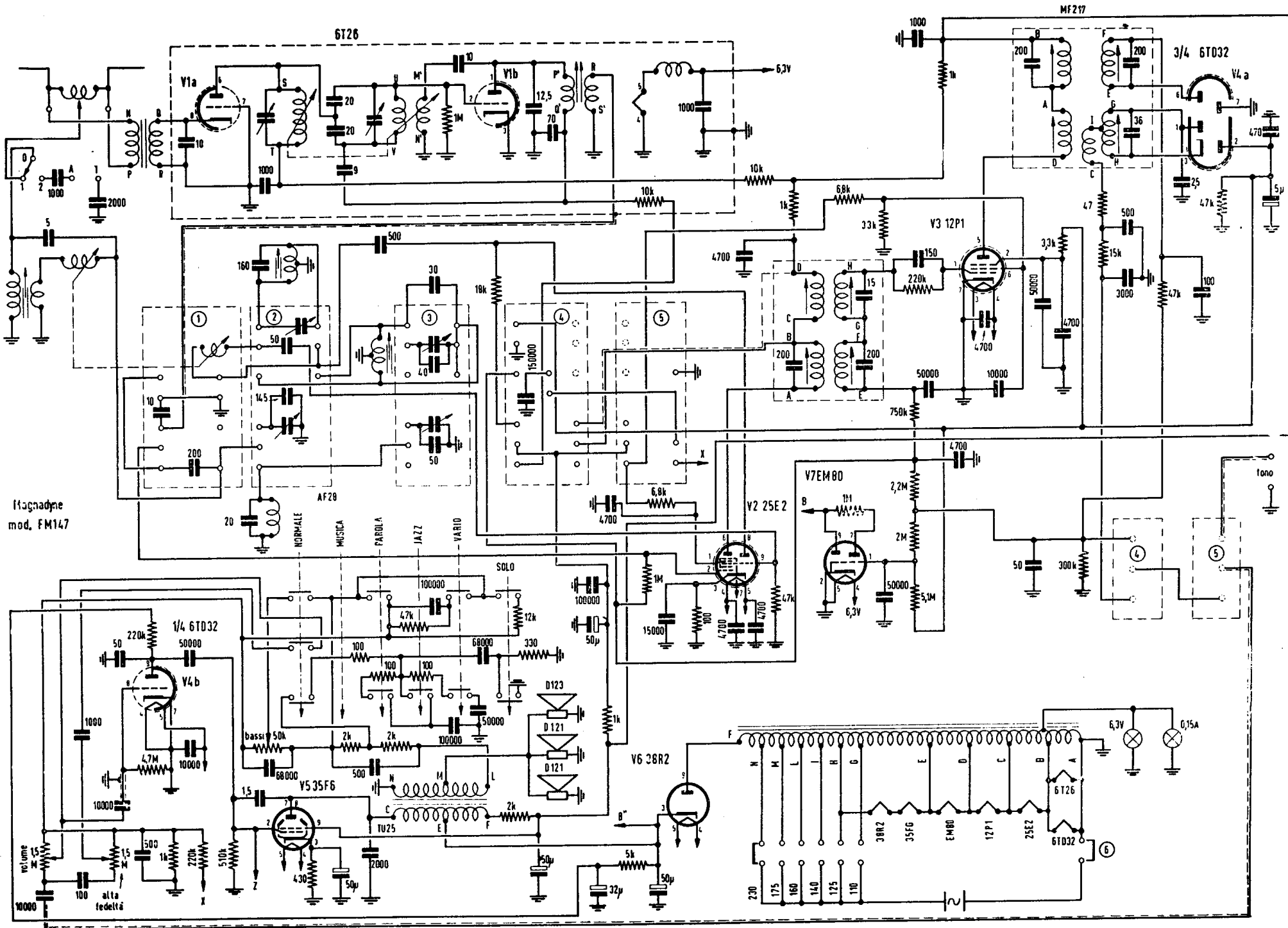
Schema elettrico del radiorecettore, Magnadyne, mod. FM 147
